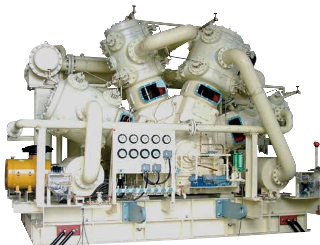
PET ブロー用オイルフリーコンプレッサ XQ3-700-OL・Pd 4.8MPa・60m³/min・730kW
